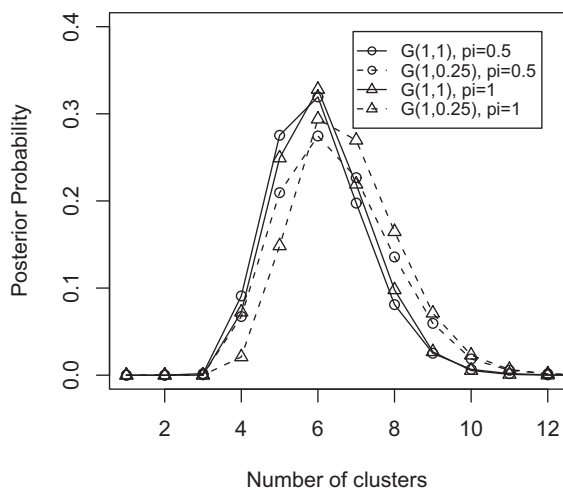
(c) Posterior number of clusters
